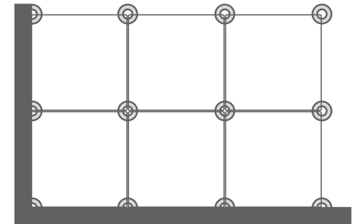
Przykładowy schemat ułożenia płyt 60x60 na wspornikach.
